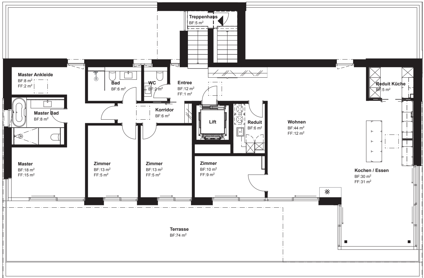
WOHNUNG 2.41 5.5-Zimmer-Wohnung Bruttfläche 204 m 2
